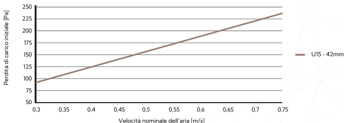
Filtro da soffitto con tenuta a gel - Codice piega: N (PH42)
