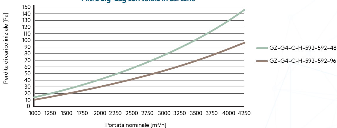
Filtro zig-zag con telaio in cartone
