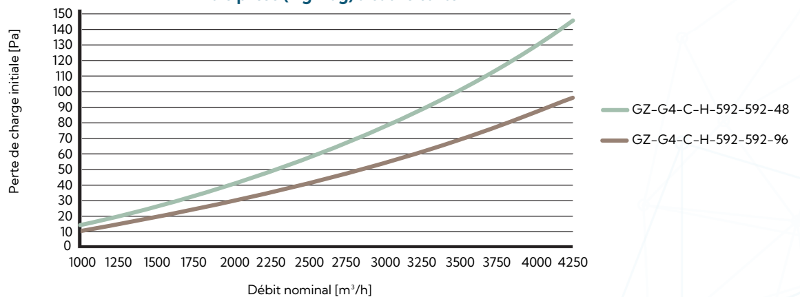
Filtre plissé (zig-zag) à cadre carton
