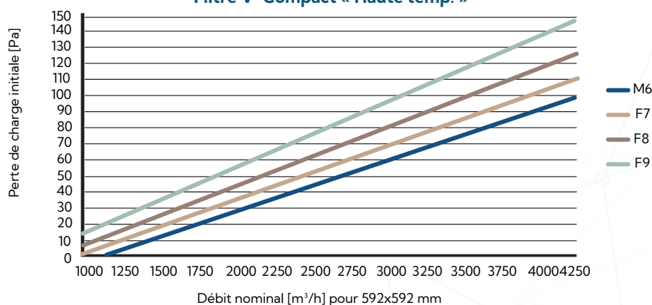
Filtre V-Compact « Haute temp. »
