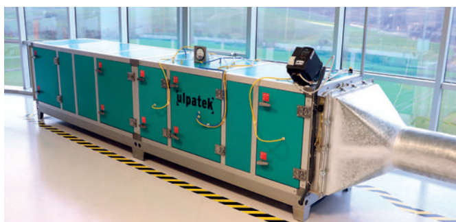
Banc d'essai de performance - PTS 5002
