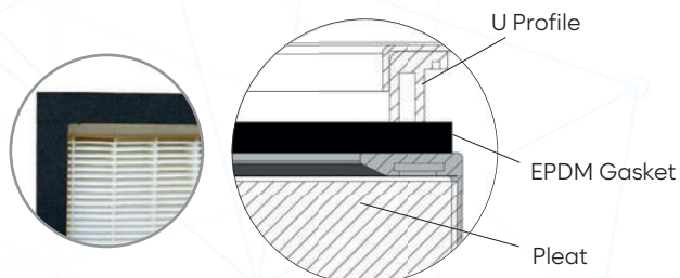
EPDM Gasket - Test Groove
