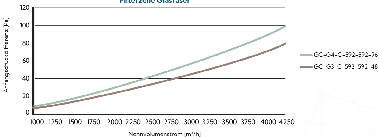
Filterzelle Glasfaser
