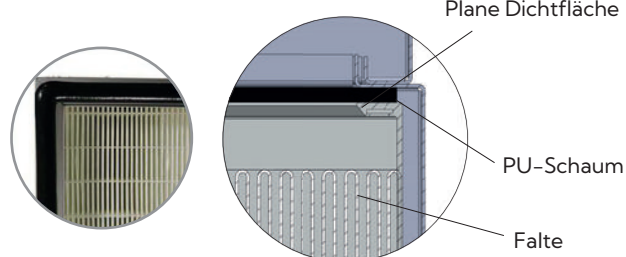
PU-Schaum – Planfläche
