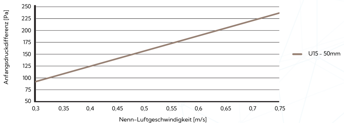
Deckenfilter mit Schneidenprofil – Faltencode: 1 (PH50)
