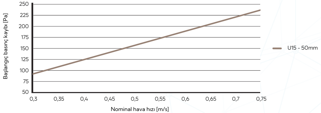
Bıçak sırtı profilili tavan tipi filtre - Pile kodu: 1 (PH50)
